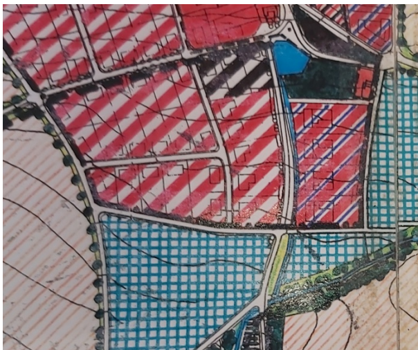
Výkres č. 2 - Funkční využití
